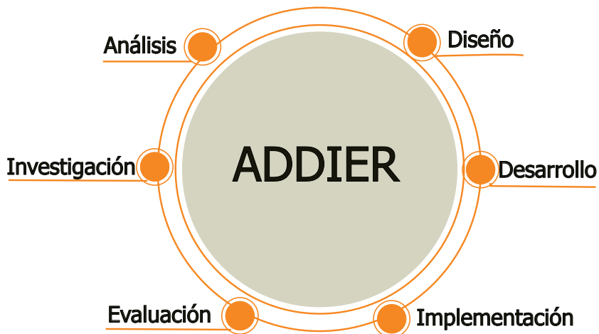
Figura 2. Modelo ADDIER.
